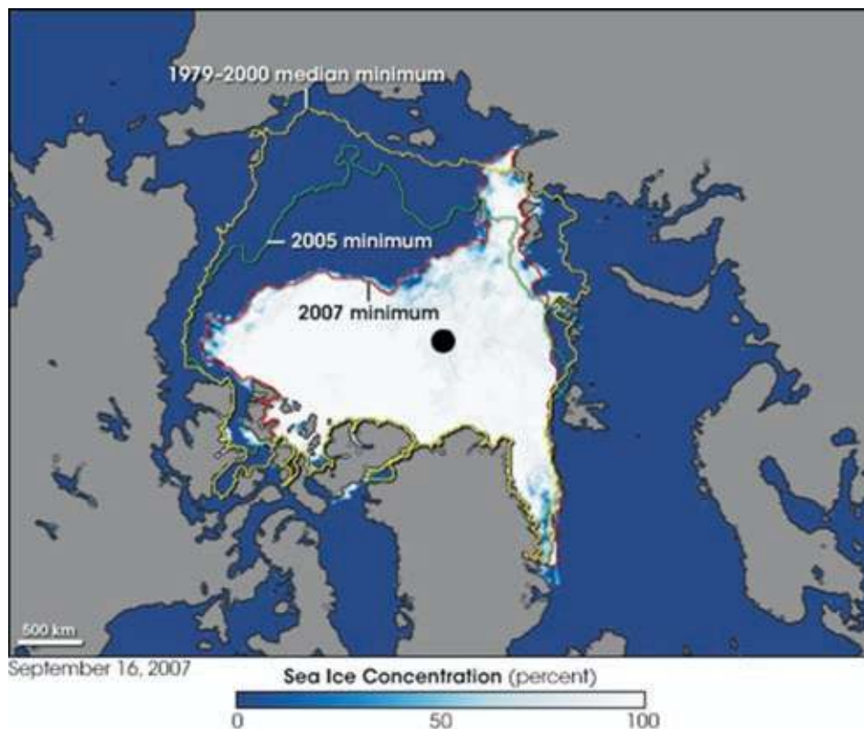
Εικόνα 2: Αυτή η εικόνα δείχνει την Αρκτική όπως παρατηρήθηκε από το Advanced Microwave Scanning Radiometer for EOS (AMSR-E) στον δορυφόρο Aqua της NASA, στις 16 Σεπτεμβρίου 2007. Η εικόνα δείχνει ένα ελάχιστο ρεκόρ των πάγων στην Αρκτική. (Πηγή: NASA, http://earthobservatory.nasa.gov/Newsroom/NewImages/images.php3?img_id=17800 )
