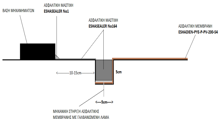
Σχέδιο 2 : Λεπτομέρεια στεγάνωσης βάσεων
