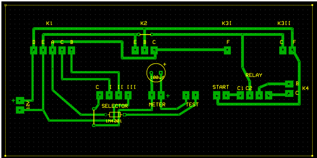
Εικόνα 4: Σχέδιο πλακέτας
